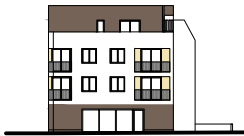
PROČELJE SJEVEROISTOK
