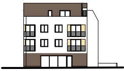
PROČELJE SJEVEROISTOK
