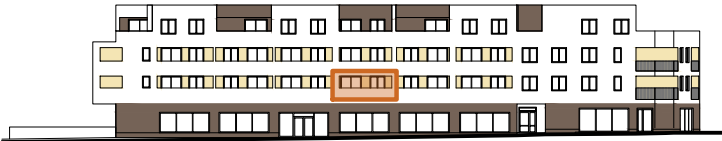
PROČELJE JUGOISTOK
